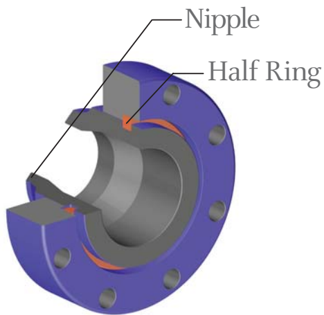
Swivel Flange Set
